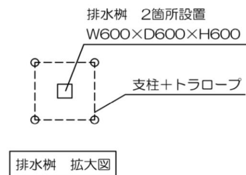
広島小屋浦油槽所跡地 排水設備（現況図）
