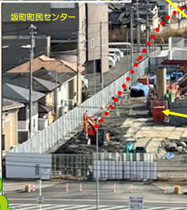
基礎杭掘削状況（U型擁壁）
