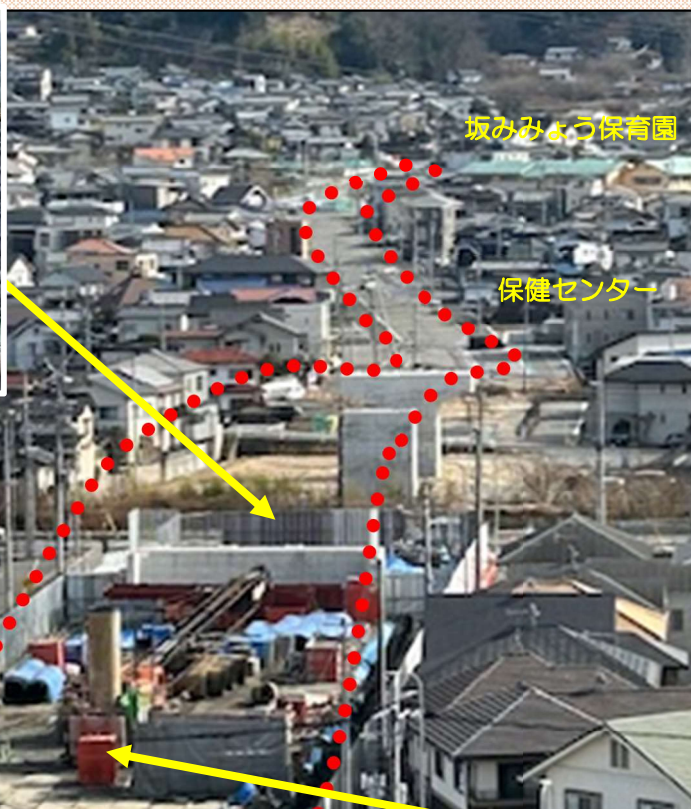
基礎杭掘削状況（U型擁壁）
