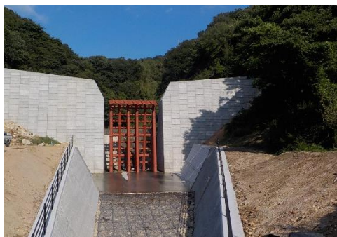
大判川（総頭山：国土交通省施工）
