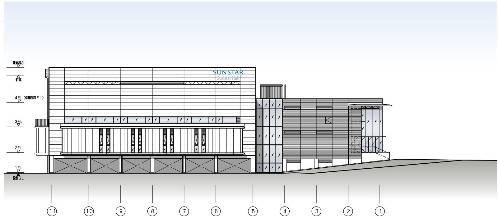
北立面图
