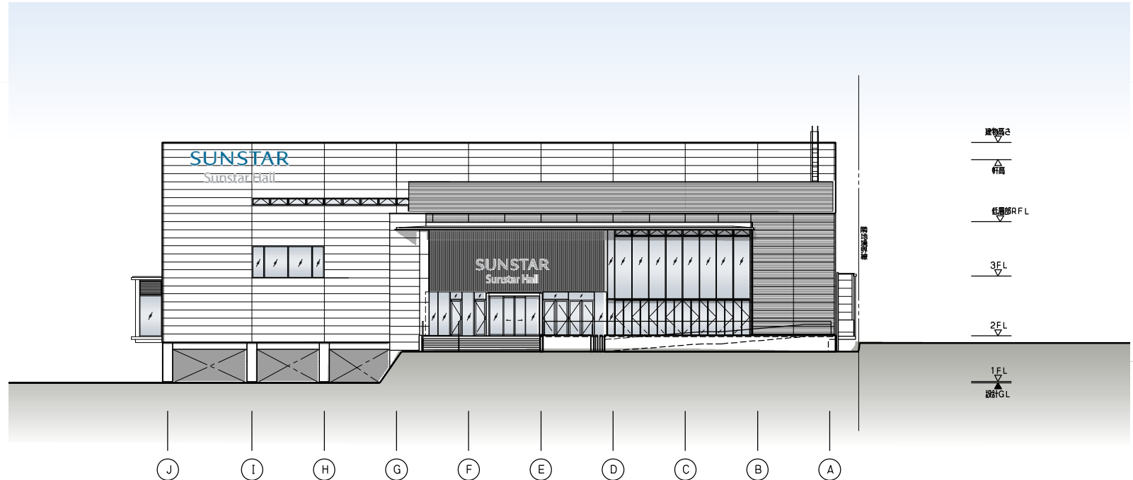
西立面图
