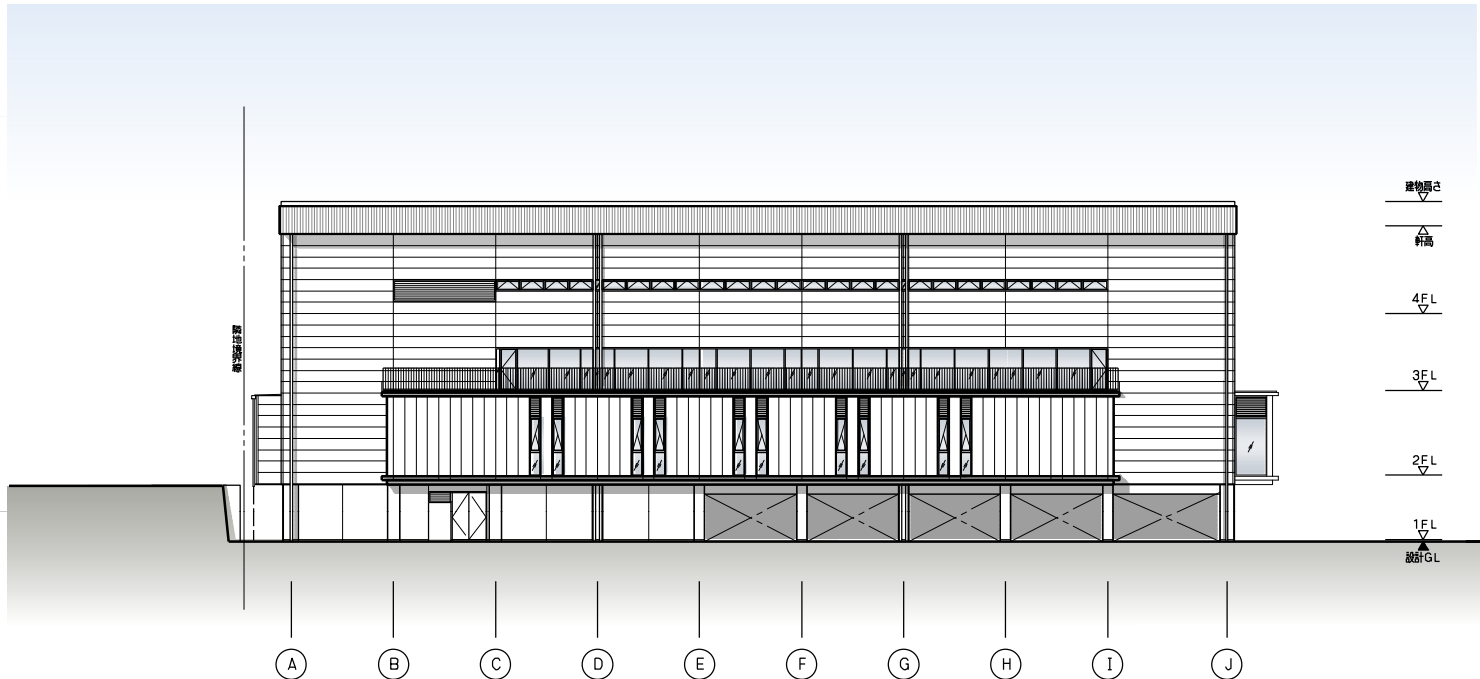
东立面图
