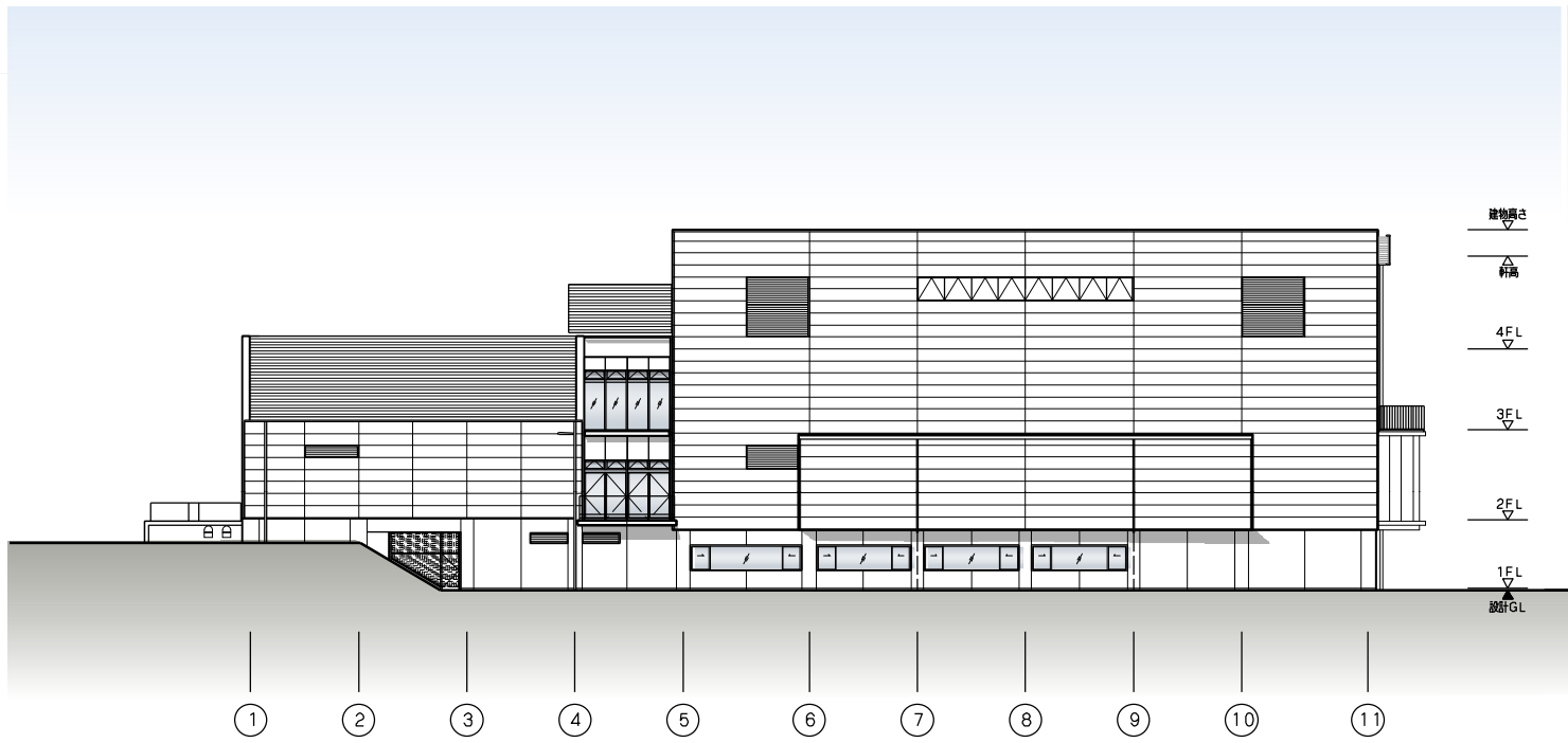
南立面图
